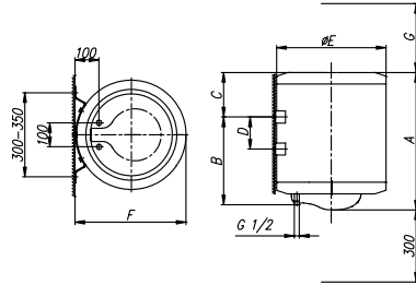
Dimensions du chauffe-eau pour le raccordement et le montage [mm]
