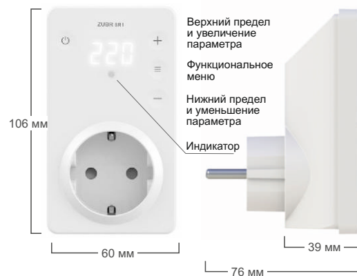
Рисунок 1. Габаритные размеры SR1
